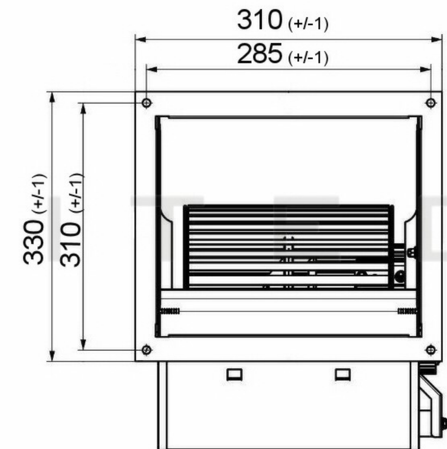
OPTIONAL EXTRA - FLANGE
